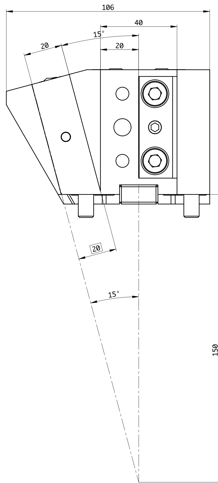
UPPER TURRET
