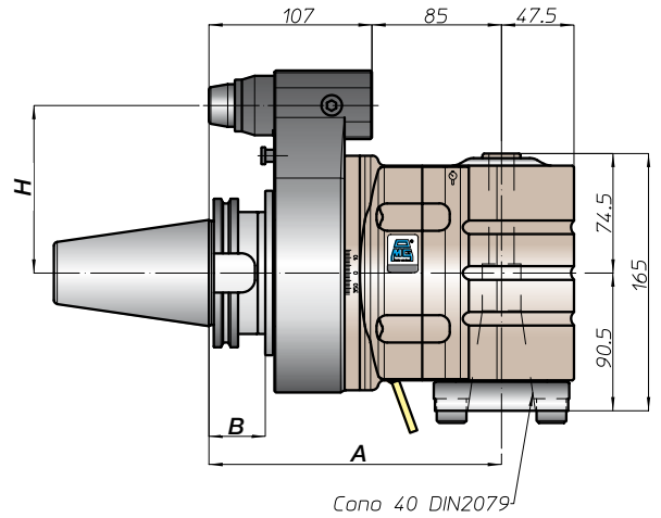
Cono 40 DIN2079
